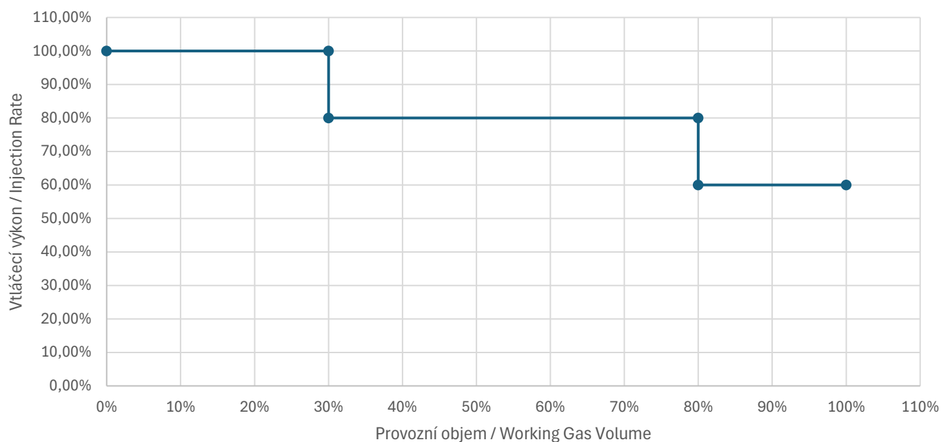
Vtláčečcí křívka / Injection Curve
