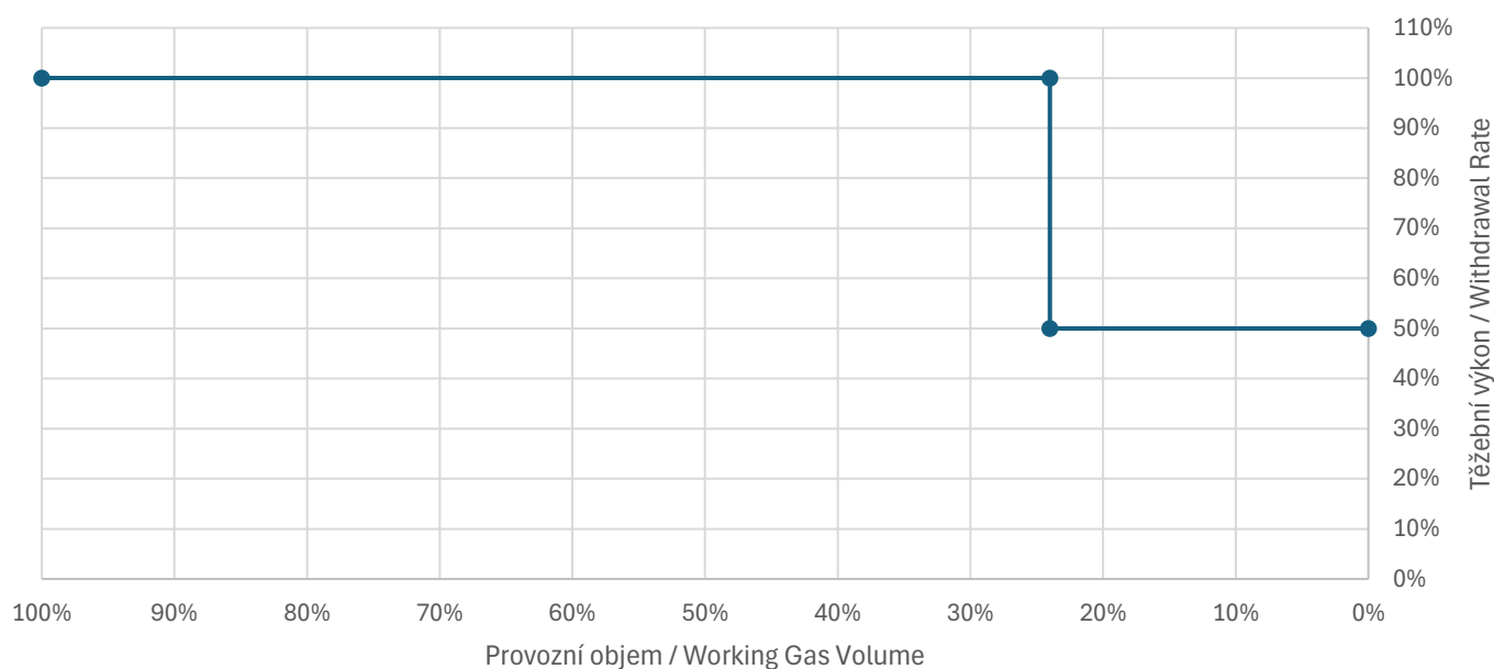
Těžečbní křívka / Withdrawal Curve
